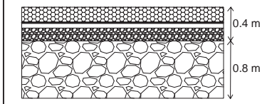
Infiltationsytå med armeringssten, överbyggnad och underliggande makadammagasin. Geotextil som materialavskiljande skikt.
