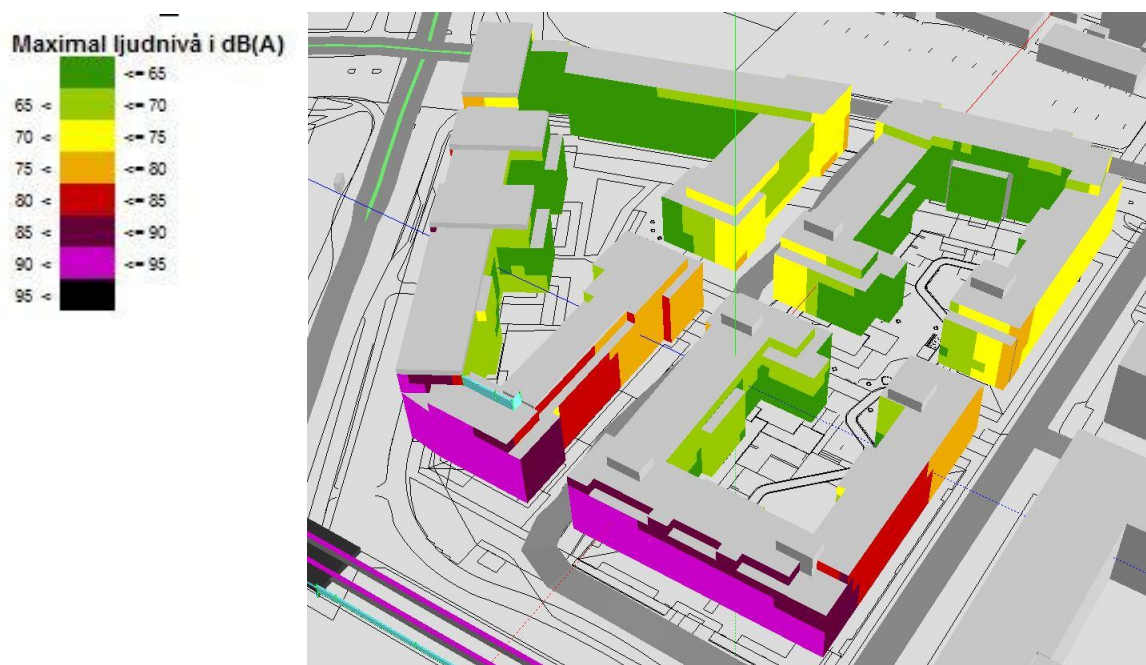
Bild 8. Maximal ljudnivå från väg- och spårtrafik. Fasader mot sydväst (mot spår och Portalgatan).
