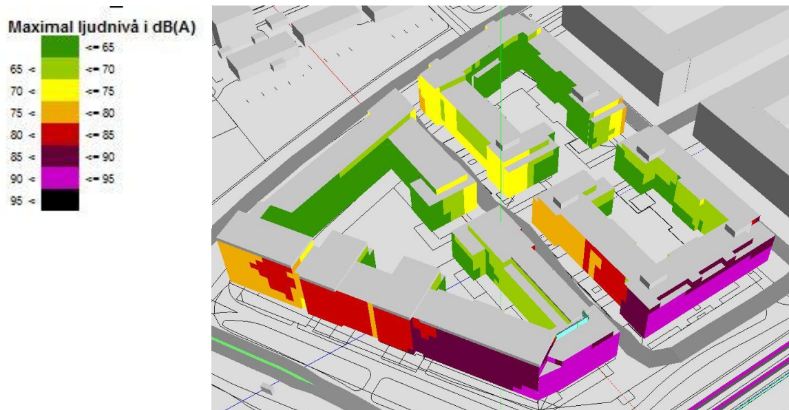
Bild 7. Maximal ljudnivå från väg- och spårtrafik. Fasader mot nordväst (mot spår och Gamla Uppsalagatan).
