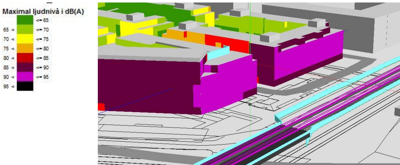
Bild 12. Maximal ljudnivå från väg- och spårtrafik med skärm längs med järnväg.
