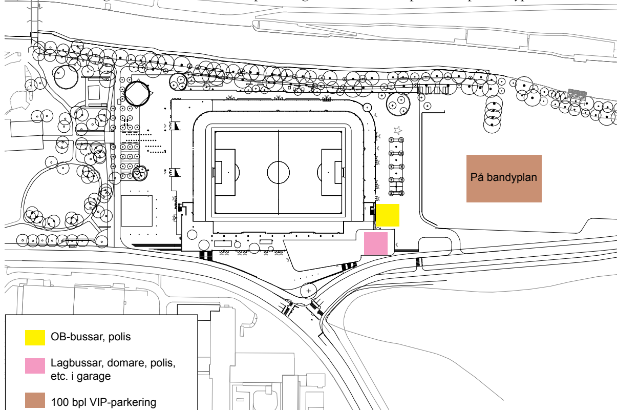
Figur 16. Parkeringsytor för domare, polis, etc. samt för lagbussar, OB-bussar och UEFAs krav på VIP-parkering
