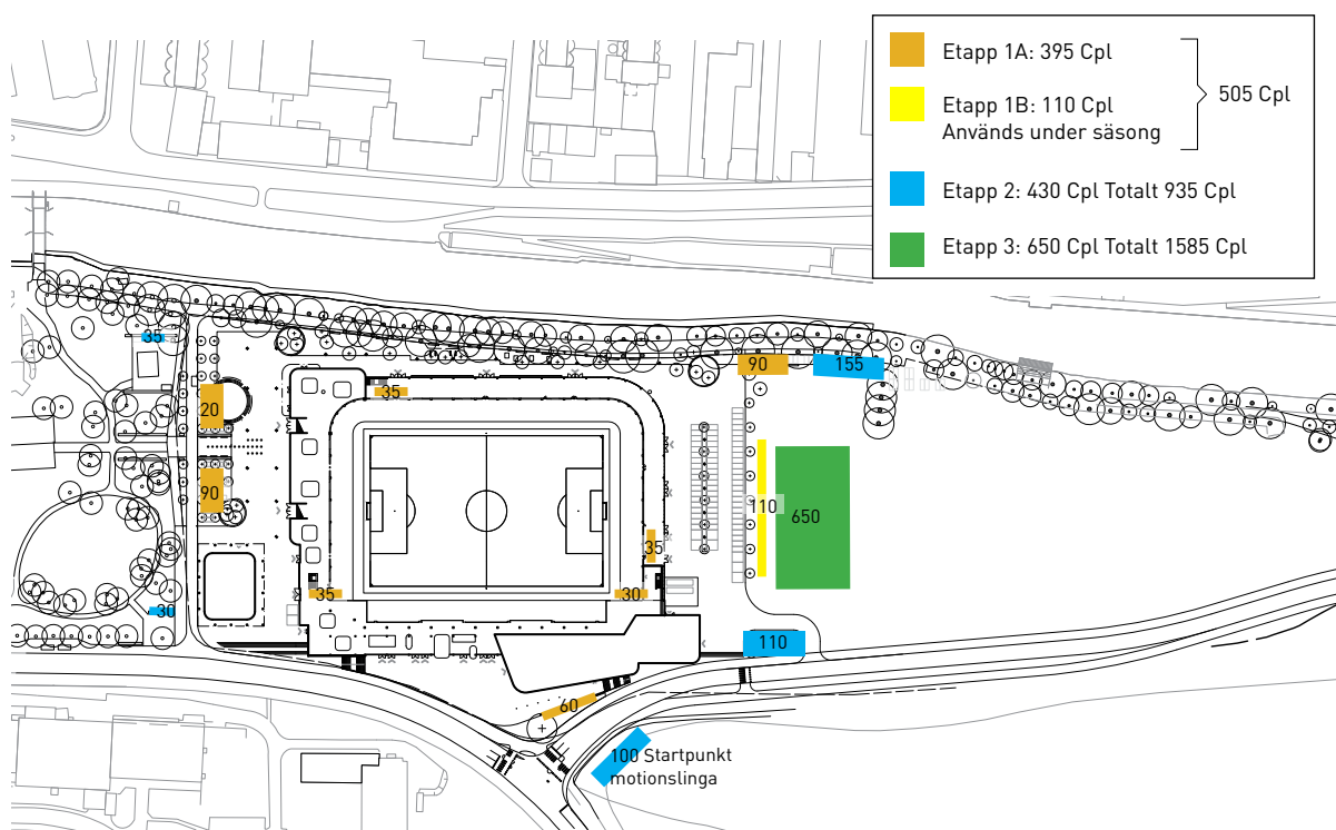
Figur 15. Föreslagen placering av cykelparkering etappvis (FOJAB 2016-07-01)
