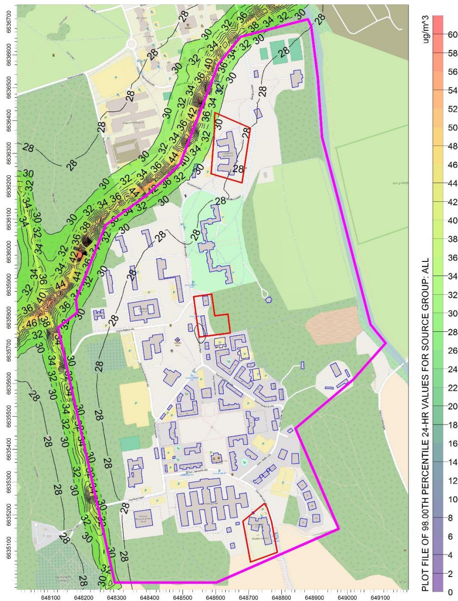
Figur 6. Nuvarande situation 2016, beräknade halter av kvävedioxid som dygnsmedelvärden. Planområdet markeras med lila linje, föreslagna byggnader med blå och skolor/förskolor med röd.
