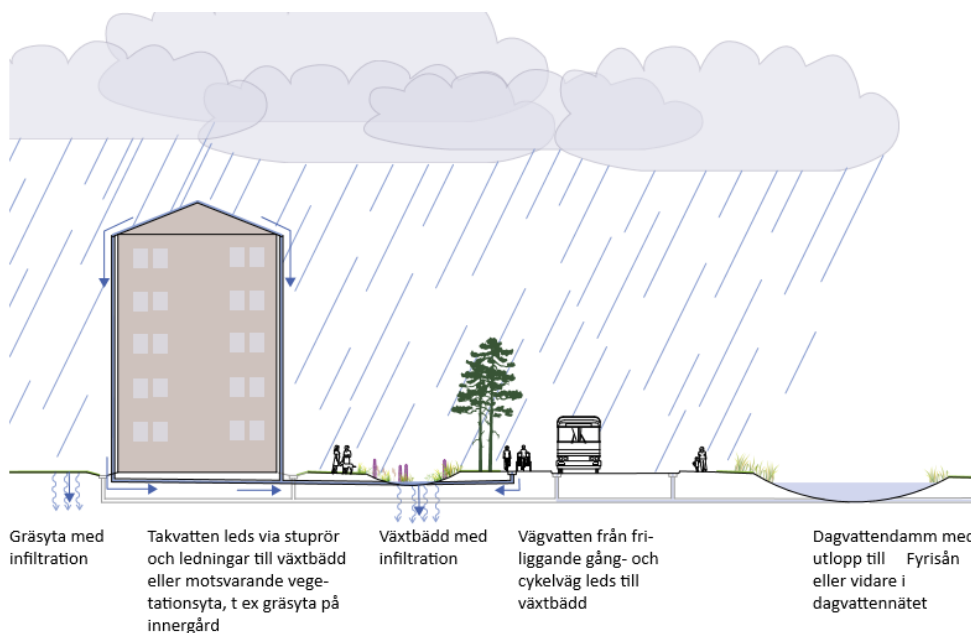
Principskiss av hantering av dagvatten från tak och gång- och cykelvägar. Illustration Bjerking.
