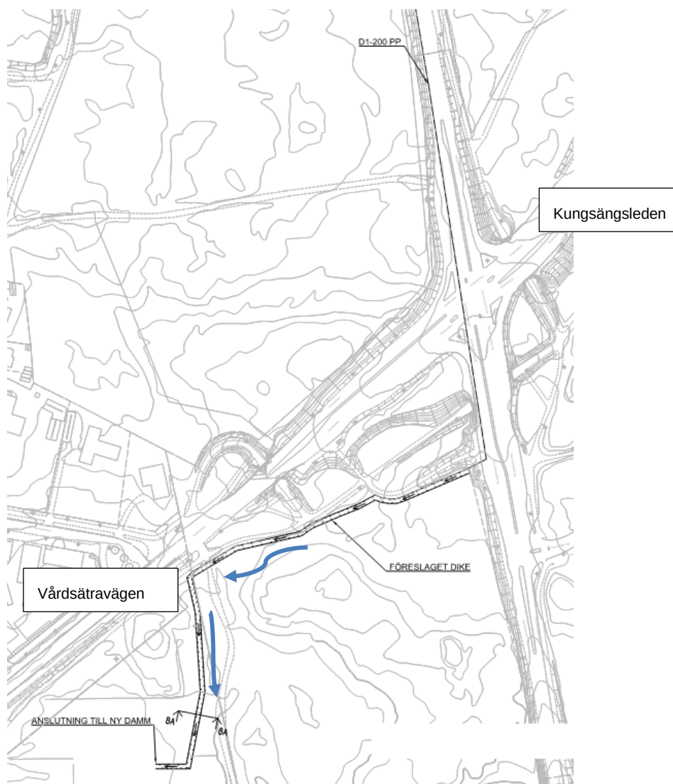
Bild 14. Alt 2 - Förslag på reningsåtgärd i makadamdike för vägdagvatten som rinner söderut till Kungsängsleden/Vårdsätravägen.
