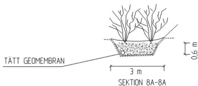
Bild 14. Alt 2 - Förslag på reningsåtgärd i makadamdike för vägdagvatten som rinner söderut till Kungsängsleden/Vårdsätravägen.
