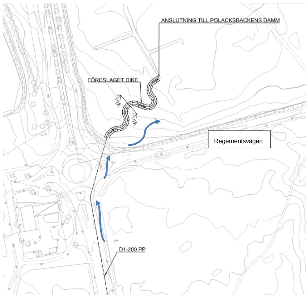
Bild 12. Alt 2 - Placering av makadamdike för vägdagvatten som rinner norrut mot Regementsvägen.
