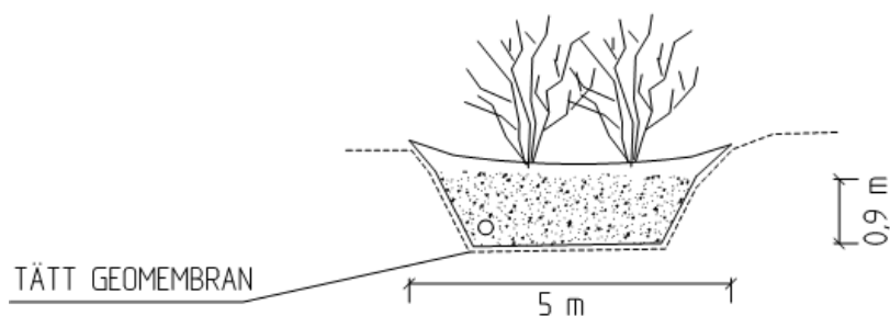
Bild 12. Alt 2 - Placering av makadamdike för vägdagvatten som rinner norrut mot Regementsvägen.
