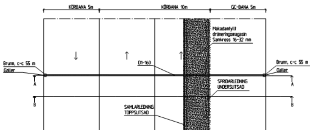
Bild 10. Alt 1 - Förslag på reningsåtgärd i makadammagasin under gång- och cykelvägen, redovisat i plan.
