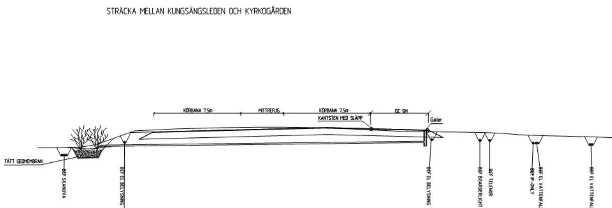
Bild 18. Förslag på reningsåtgärd i växtbädd redovisat i sektion C-C.
