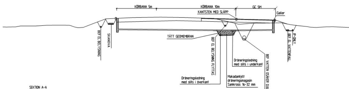
Bild 11. Alt 1 - Förslag på reningsåtgärd i makadammagasin under gång- och cykelvägen, redovisat i sektion A-A.
