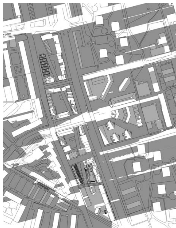
VÅR OCH HÖSTDAGSJÄMNING KL17
