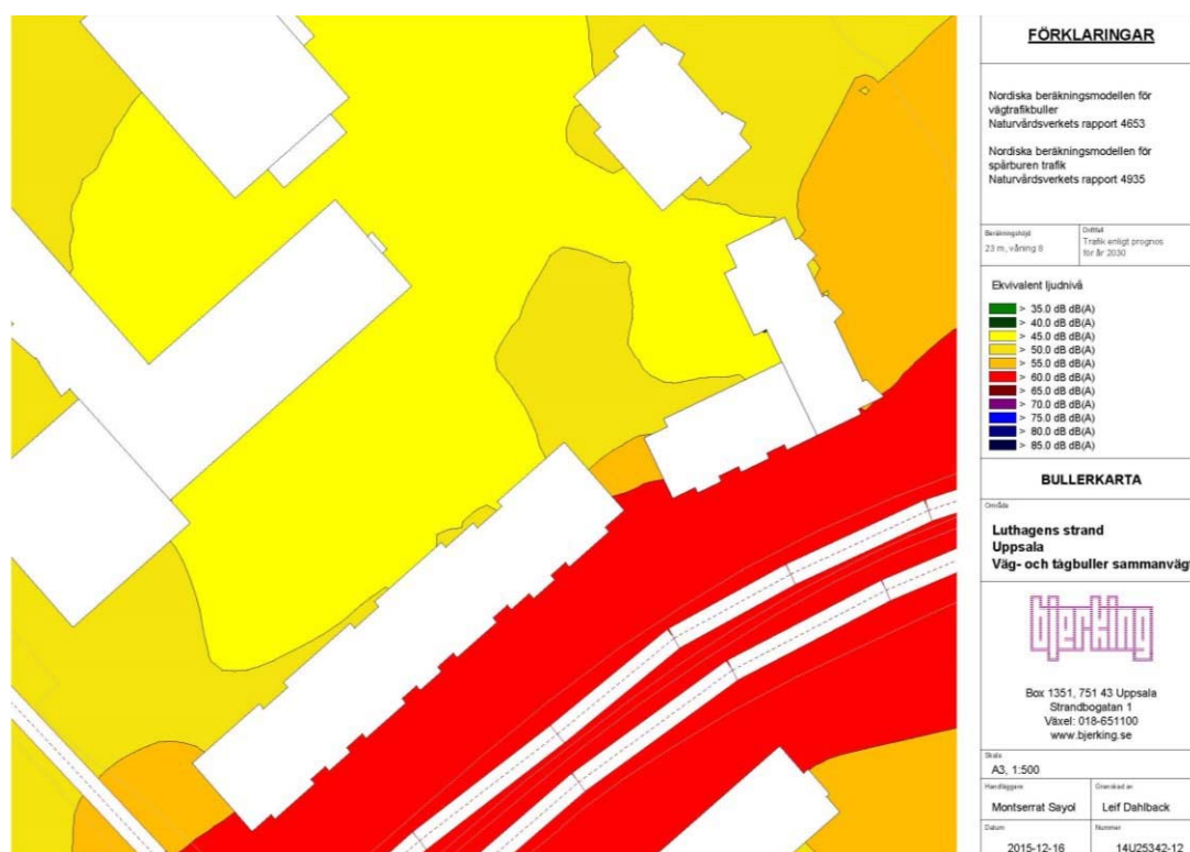
Ekvivalenta ljudnivåer vid 40 km/h, våning 8, 23 meter ovan mark, Björking.
