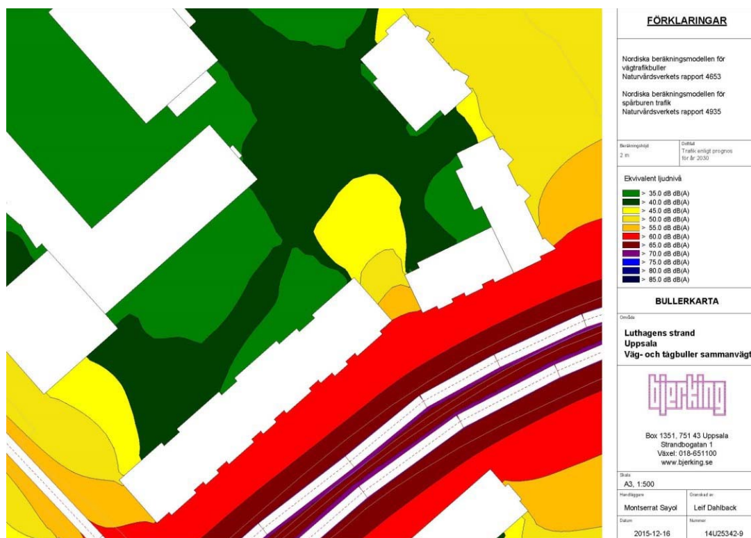
Ekvivalenta ljudnivåer vid 40 km/h, två meter ovan mark, Björking.
