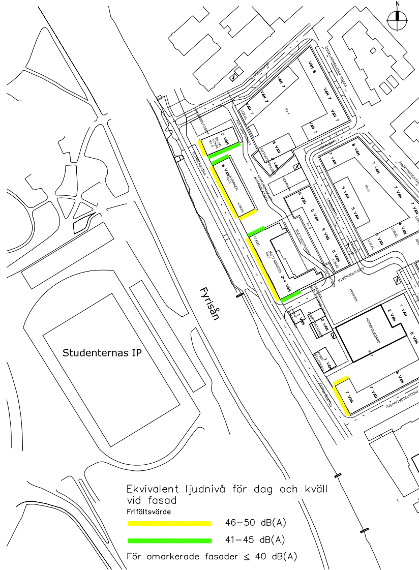
Situationsplan. Ljud från idrottsplats. Ekvivalentnivåer vid fasad. (Bullerutredning, ÅHA, 2018)
