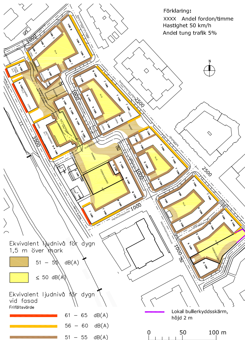
Situationsplan. Ljud från trafik. Ekvivalentnivåer vid fasad och över mark. (Bullerutredning, ÅHA, 2018)
