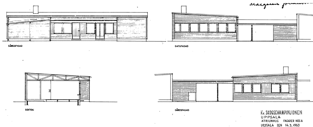
Fasadritningar av byggnadernas i ursprungligt uppförande.
