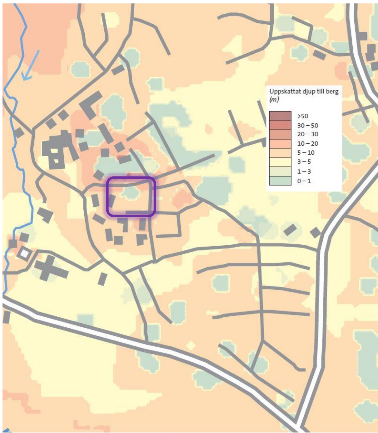
Figur 3-4. Jorddjupet för planområdet fastighet 1:51 Bålinge.
