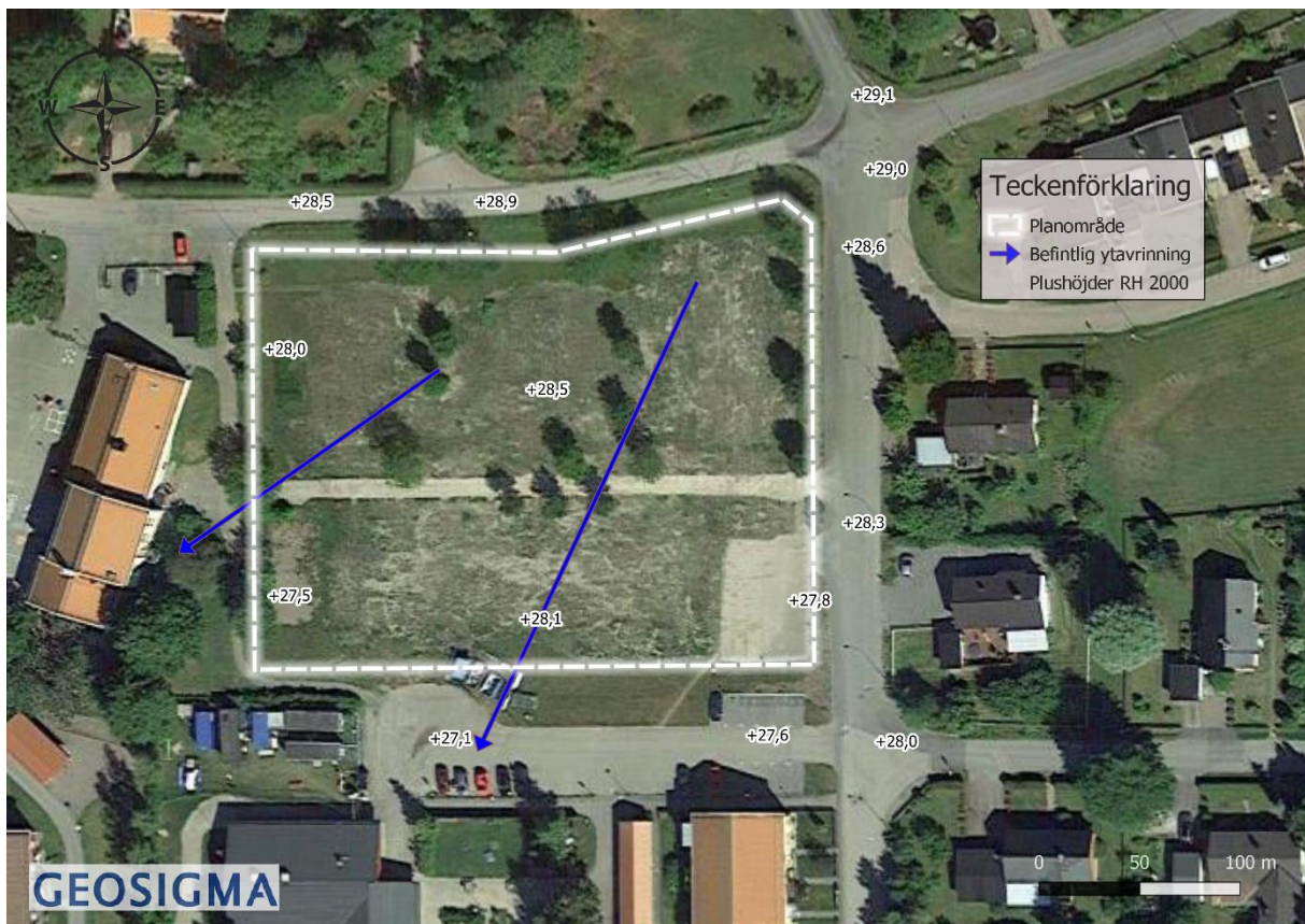
Figur 3-5. Ytavrinning, enligt befintlig markanvändning, inom planområdet som sluttar lätt åt sydväst.
