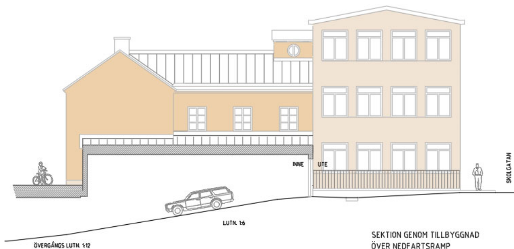
11 Sektion över nedfart till underjordiskt garage. Illustration Fidjeland och Partners Arkitekter AB.
