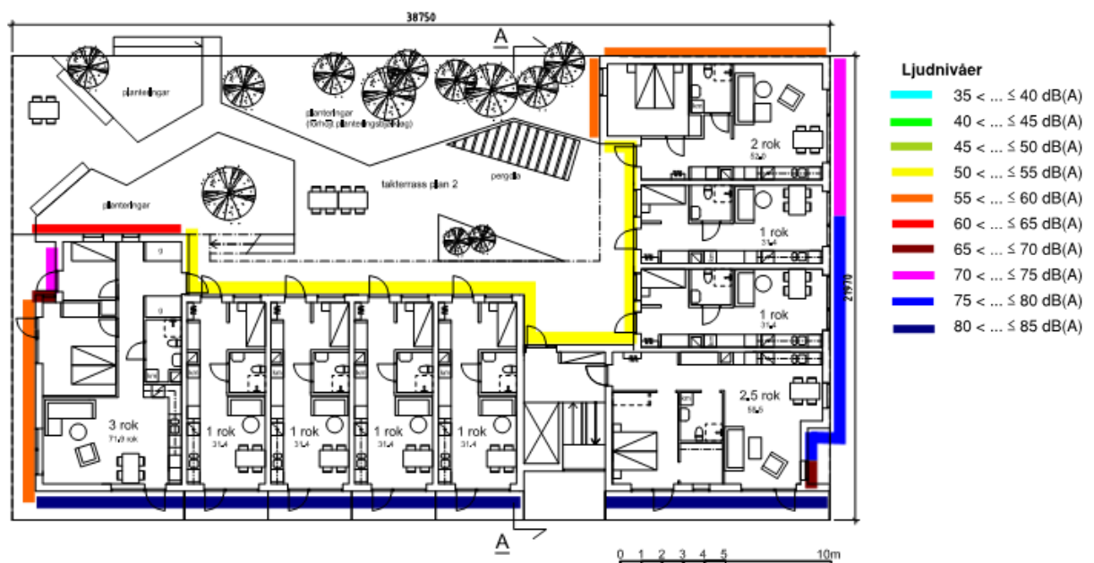
Figur 2. Maximal ljudnivå vid fasad plan 2
