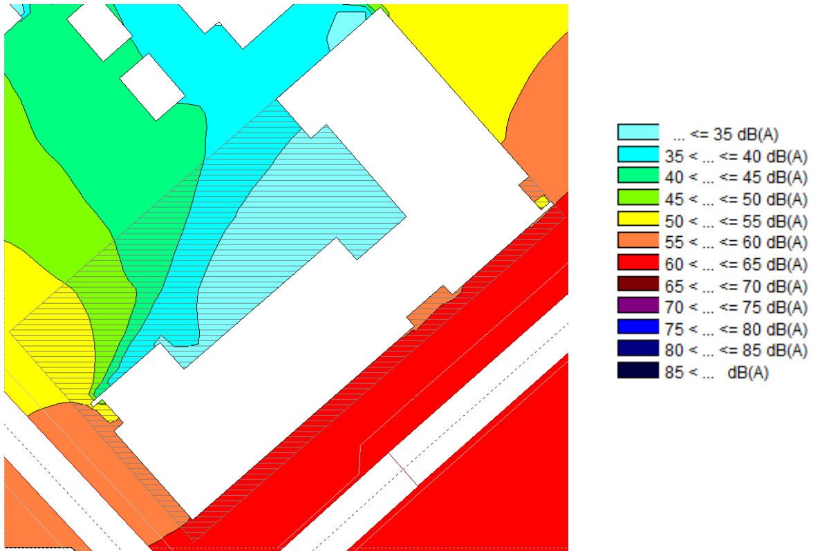
Figur 3. Ekvivalent ljudnivå takterrass plan 2
