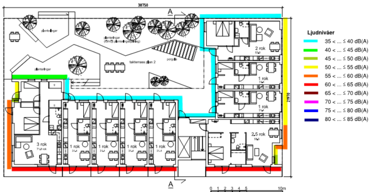
Figur 1. Ekvivalent ljudnivå vid fasad plan 2.
