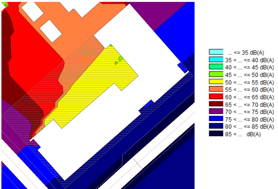
Figur 4. Maximal ljudnivå takterrass plan 2
