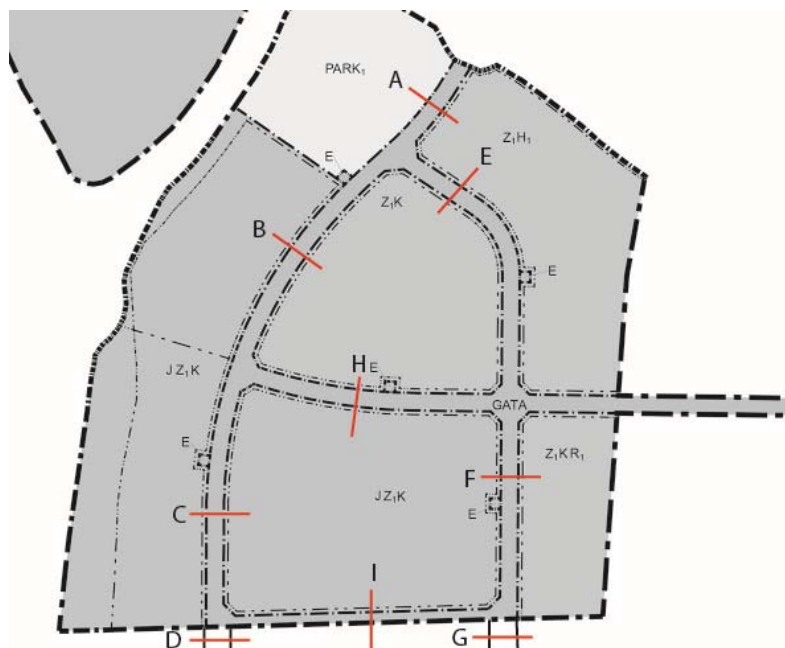
Beräknade trafikmängder vid ett fullt utbyggt område, fordon/dygn (ÅDT) och trafikmängd tung trafik (ÅDT tung). Andelen tung trafik bedöms vara 15 %.
