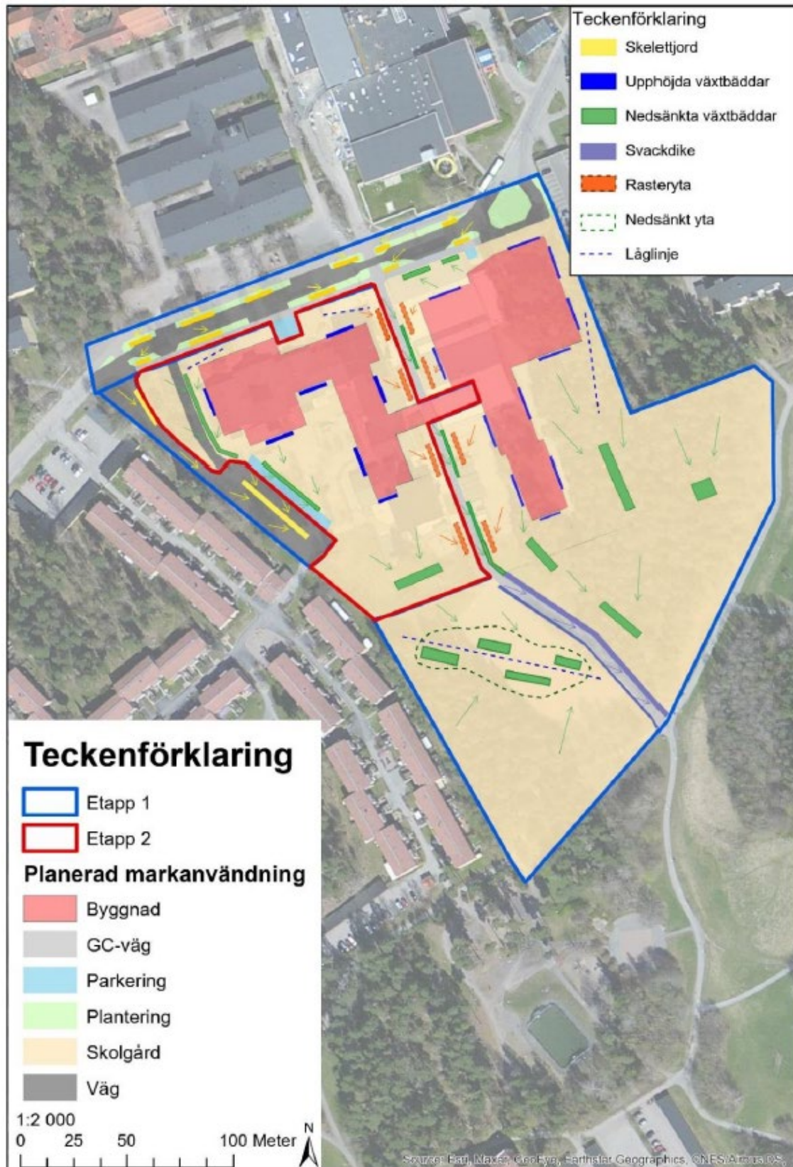
Figur 21 Utdrag ur dagvattenutredning. Kartan visar hur dagvattenhantering kan utföras. Lösningen är baserad på förslaget från steg 2. (WSP)
