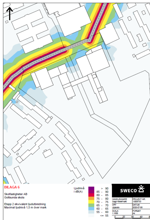
Figur 30 Utdrag ur trafikbullerutredning. Maximal ljudutbredning och ljudnivå 1,5 meter över mark. (Sweco)
