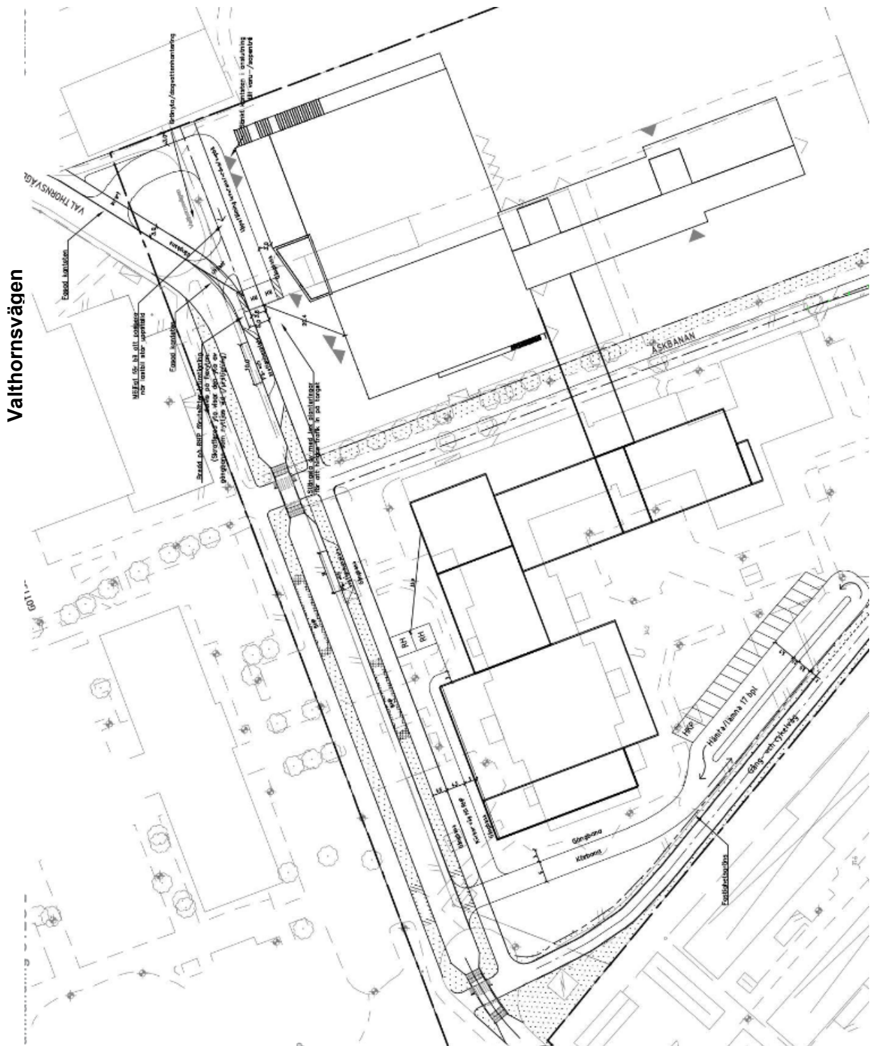
Figur 28 Situationsplan som visar trafiklösningen. (Cedervall Arkitekter)
