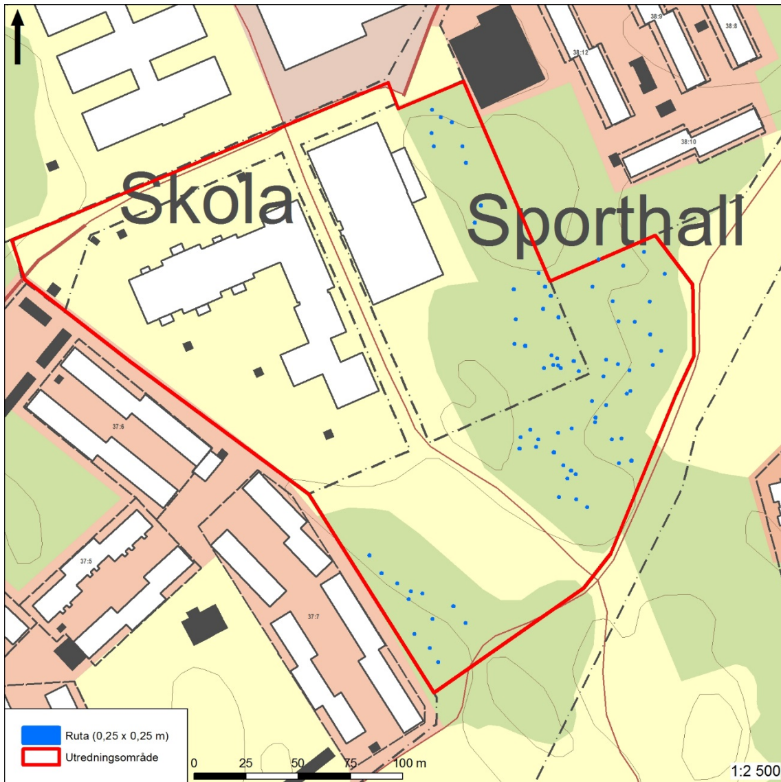
Figur 1. Resultatplan som visar provrutorna (blått) och utredningsområdet (rött) med fastighetskartan som bakgrund. Skala 1: 2 500.
