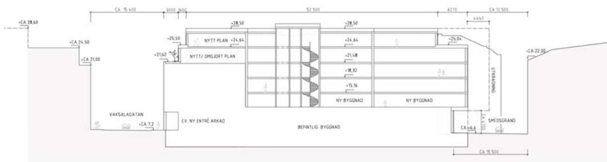
SEKTION B-B
