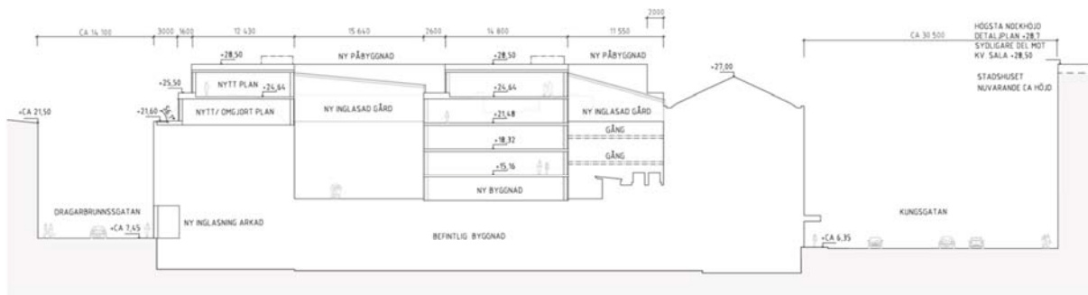
SEKTION A-A
