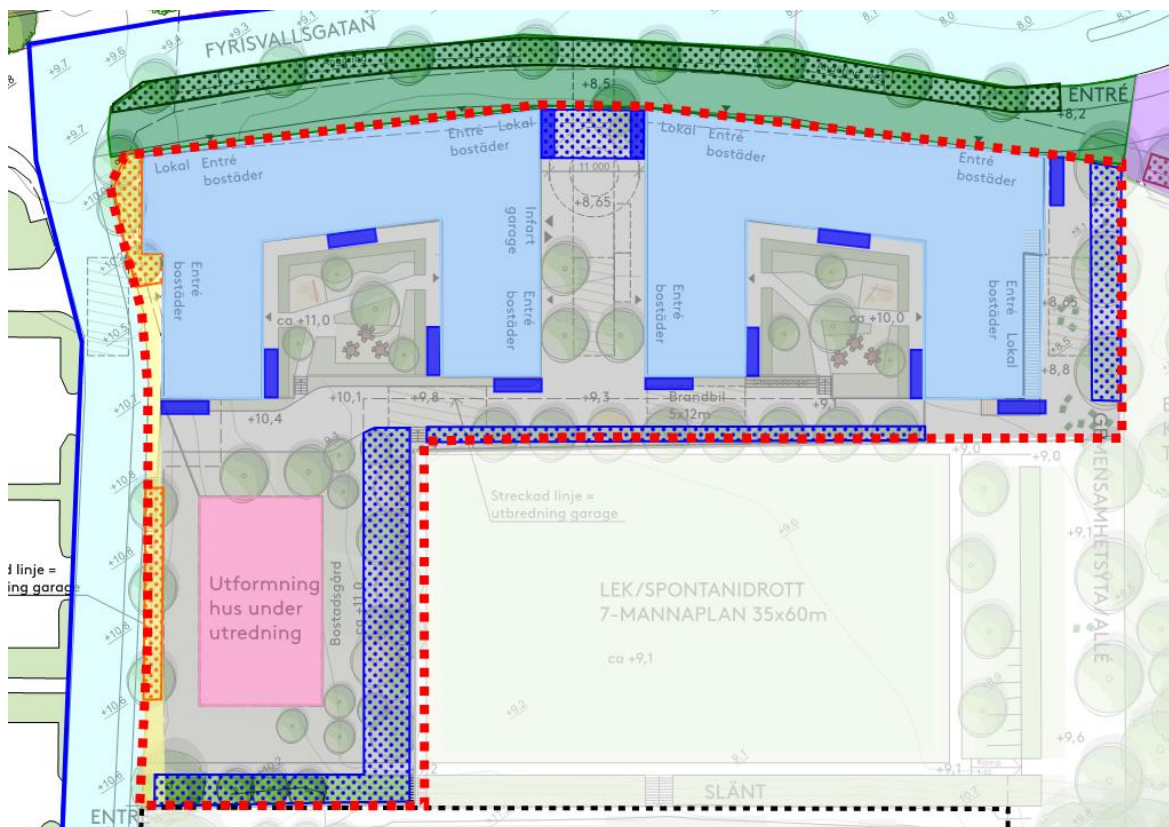
Figur 3-2. Åtgärdsförslag dagvattenhantering inom område för ny bebyggelse.
