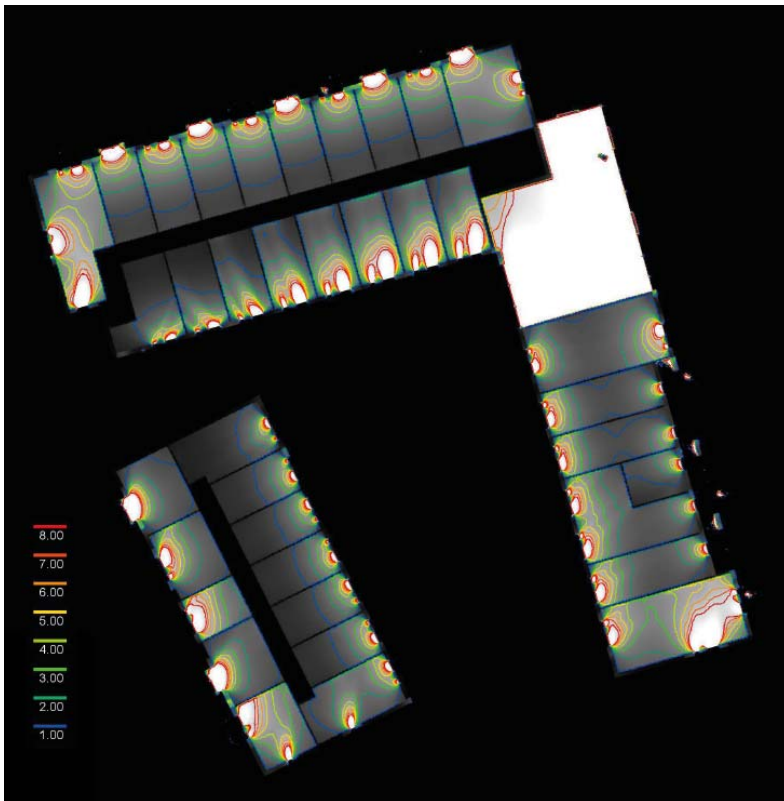
Dagsljusanalys för nedersta bostadsplanet. Kravet är att det område som begränsas av blå linje (dagsljusfaktor 1,0) ska täcka minst halva bostadsytan exklusive badrum etc.
