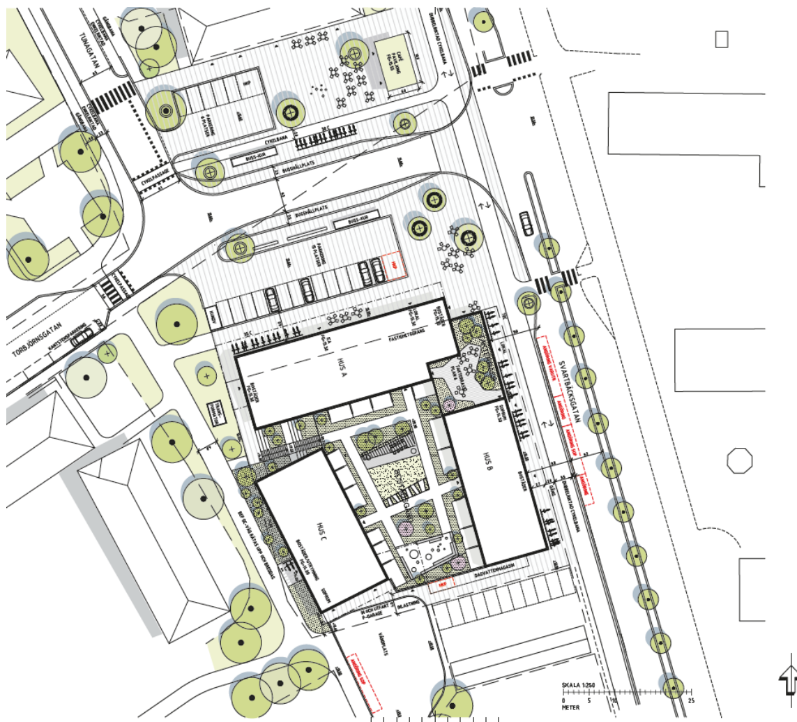
Situationsplan. I samband med byggnationen flyttas busshållplatserna till Torbjörns torg och på torget skapas fler vistelsezoner. Karavan & SustainVR.
