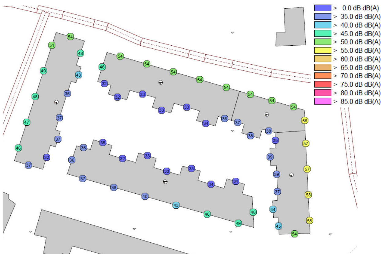
Kartan visar de ekvivalenta bullernivåerna vid fasad på våning 1. Kvarteret är mest bullerutsatt mot Hildur Ottelinsgatan i öster.
