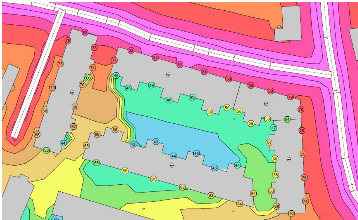
Kartan visar de maximala bullernivåerna vid fasad, 2 meter över mark.
