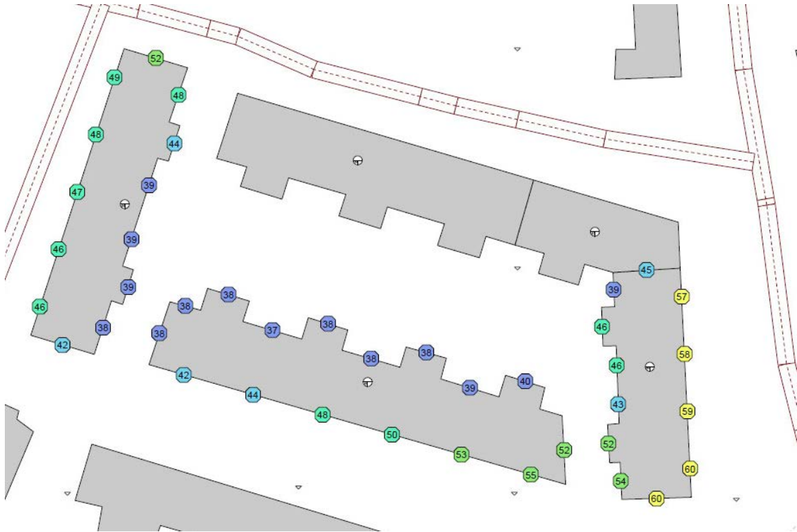
Kartan visar de ekvivalenta bullernivåerna vid fasad på våning 5. Kvarteret är mest bullerutsatt mot Hildur Ottelingsgatan i öster och de övre våningsplanen har de högst värdena.
