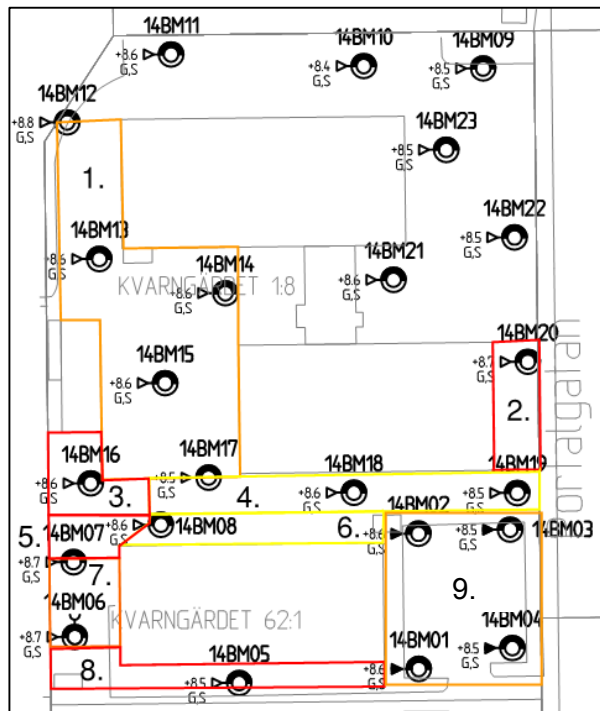
Figur 2. Uppskattad utbredning av föroreningar uppdelad på olika föroreningshalter där gult visar på halter mellan KM och MKM, orange på halter mellan MKM och farligt avfall och röd på halter över farligt avfall.
