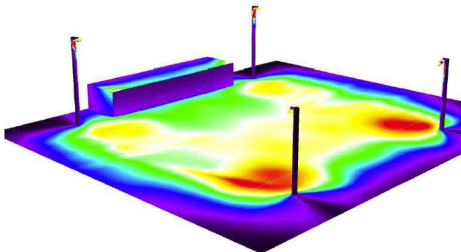
Illustration av belysningsstolpar och en grov volymskiss av den nya föreslagna läktarbyggnaden.
