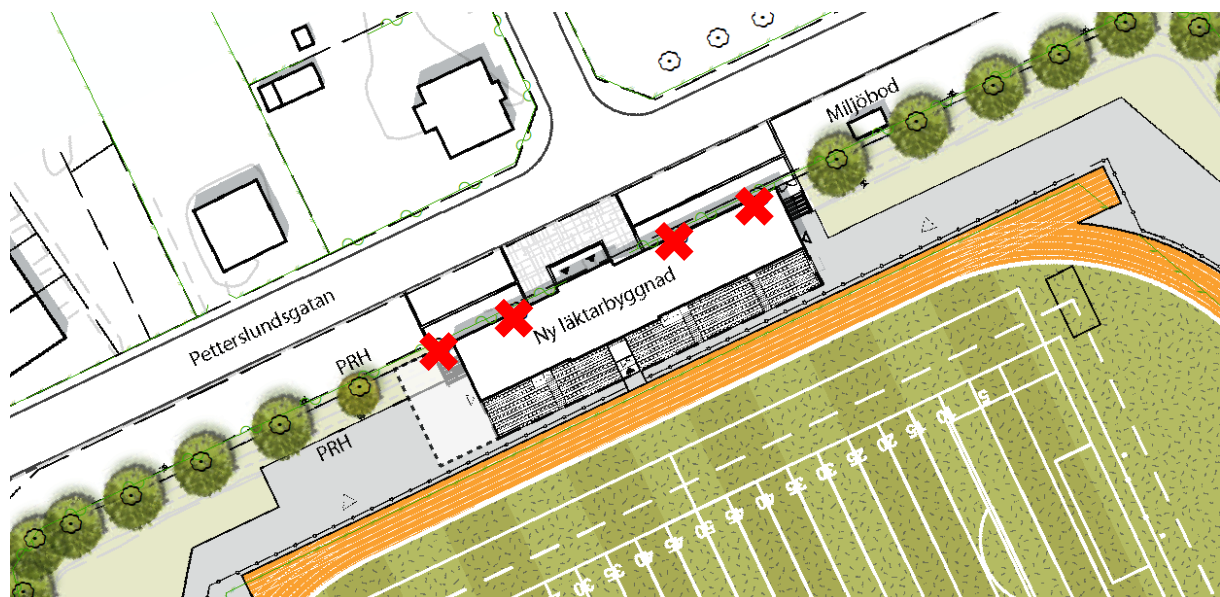
Illustration av ett förslag på ny läktarbyggnad som möjliggörs på Österängens IP. För att möjliggöra ett av de mer utbyggda scenarierna för den nya läktaren behöver preliminärt 4 lönnar tas bort (markerade med röda kryss).
