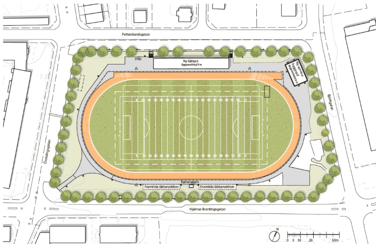
Situationsplan över ett förslag på utbyggnad av Österängens IP som möjliggörs. I illustrationen ovan visas ett exempel där de biotopskyddade träden blir kvar.
