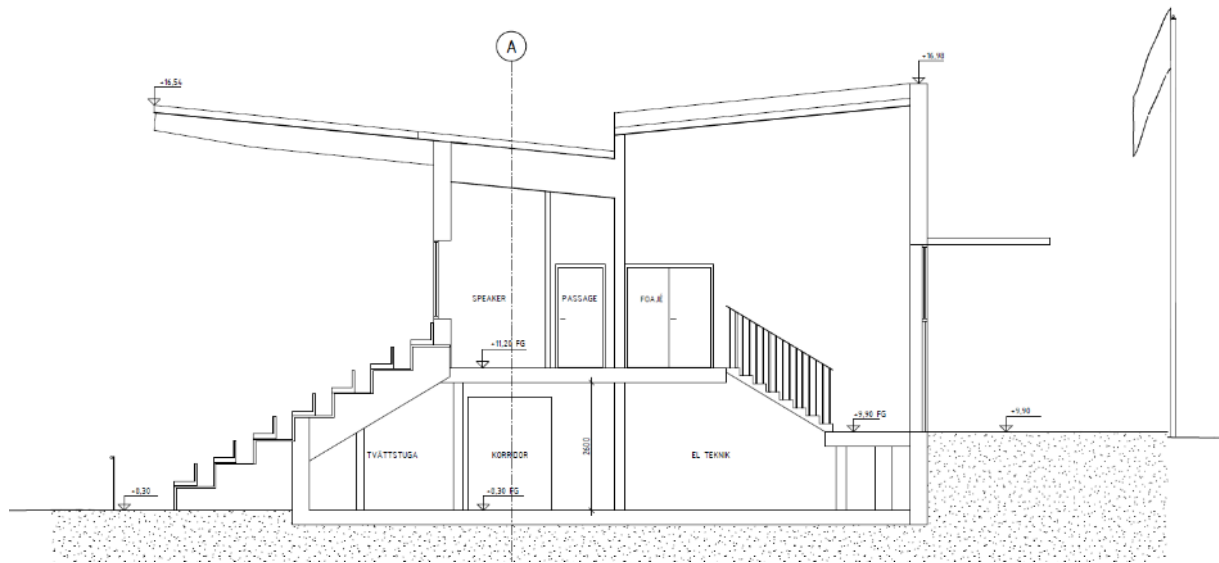
Sektionsskiss på den typ av läktarbyggnad som möjliggörs mot Petterslundsgatan (entré mot gatan till höger).
