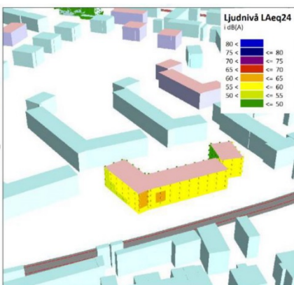
Fasadljudnivåer, ny byggnad längs Luthagsesplanaden.
