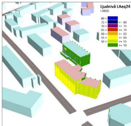
Fasadljudnivåer, ny byggnad längs S:t Johannesgatan.
