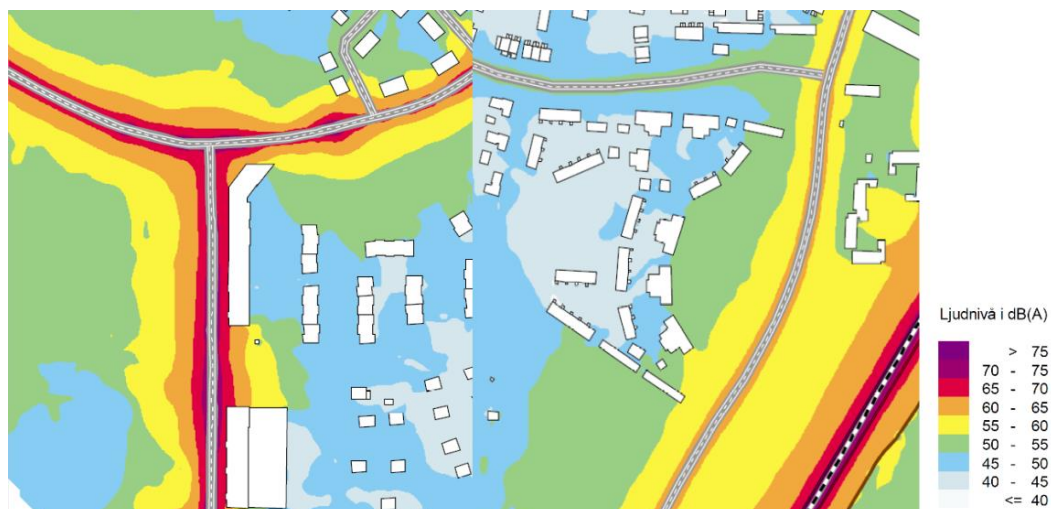
Figur 15. Ekvivalent ljudnivå vid befintlig bebyggelse i söder vid Norra Fullerö hage (till vänster) och i norr vid Åskmolnsvägen (till höger).
