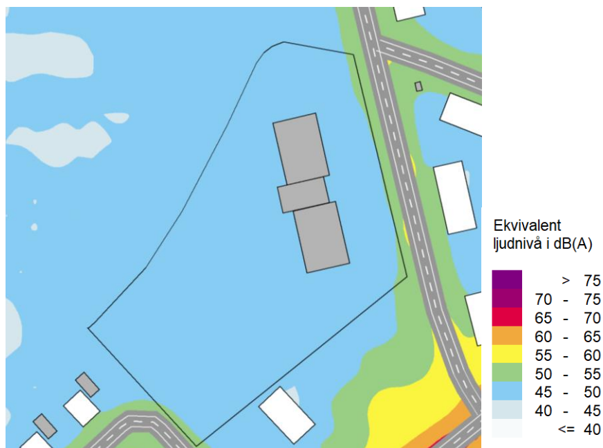
Figur 6. Ekvivalent ljudnivå över yta för förskola, prognosår 2040. Mark för förskolegård är inringad i svart.
