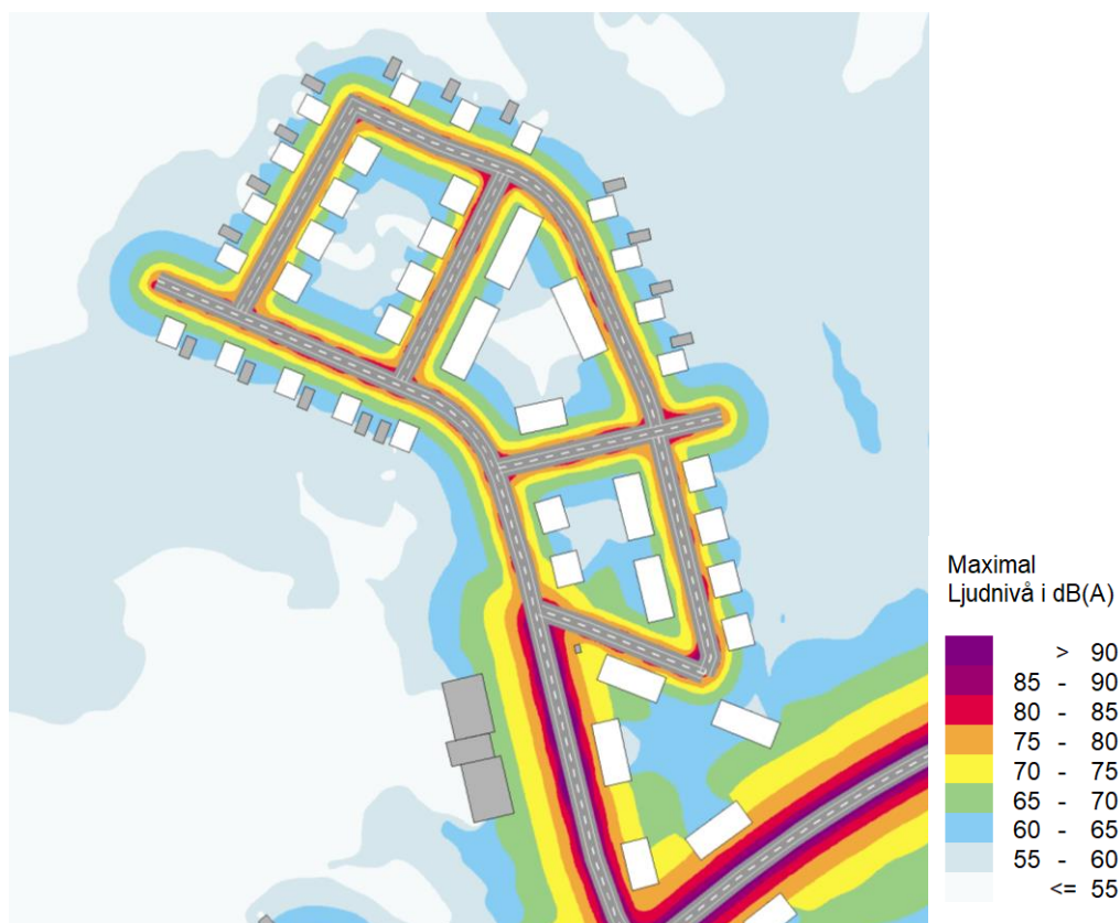
Figur 12. Maximal ljudnivå på uteplatser prognosår 2040, delområde B.
