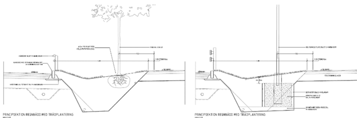
Principsektioner av regnbäddar för dagvattenhantering längs Kungsängsesplanaden (Ramböll).
